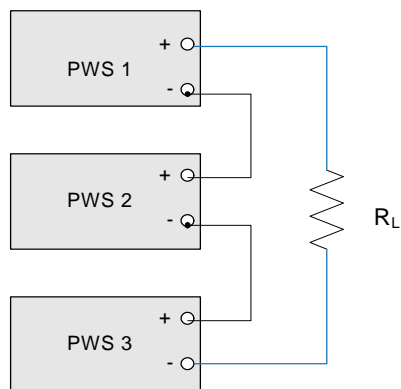
串联设置
