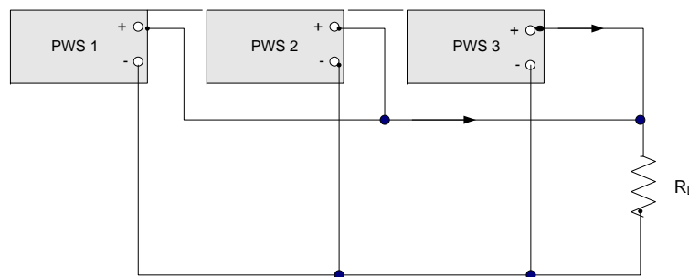
并联设置
